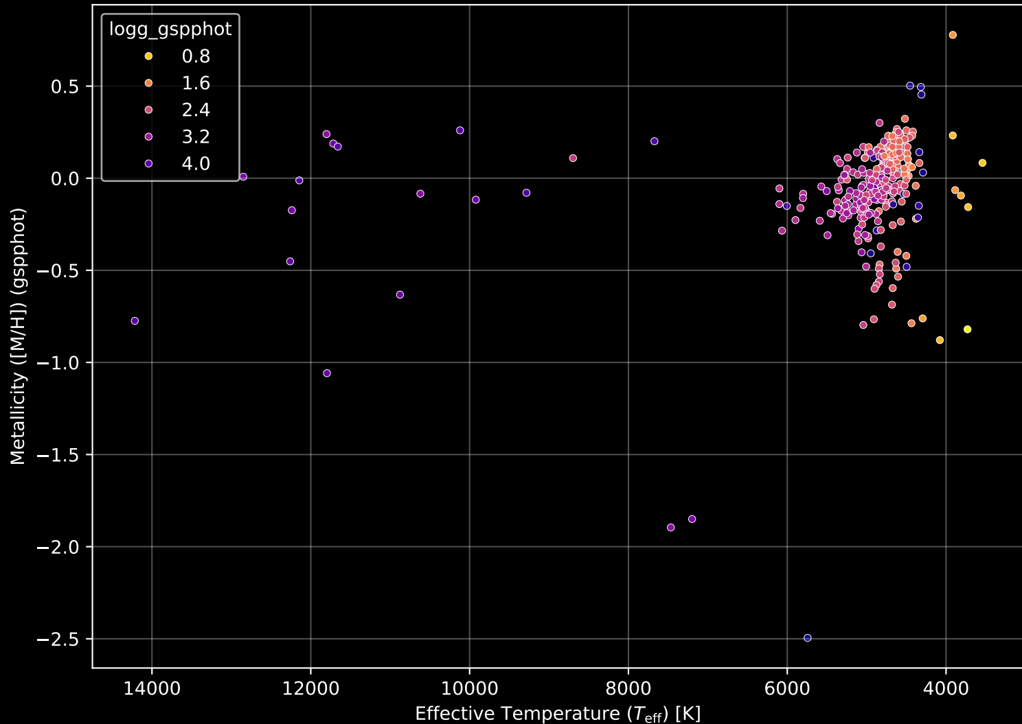
APOGEE DR17 Field: [140-06] Stellar Population Parameters (n= 325)
